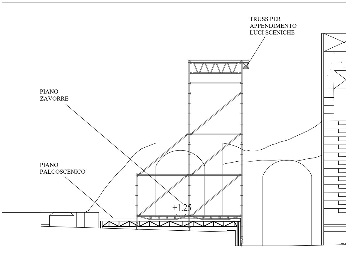
VISTA LATERALE
