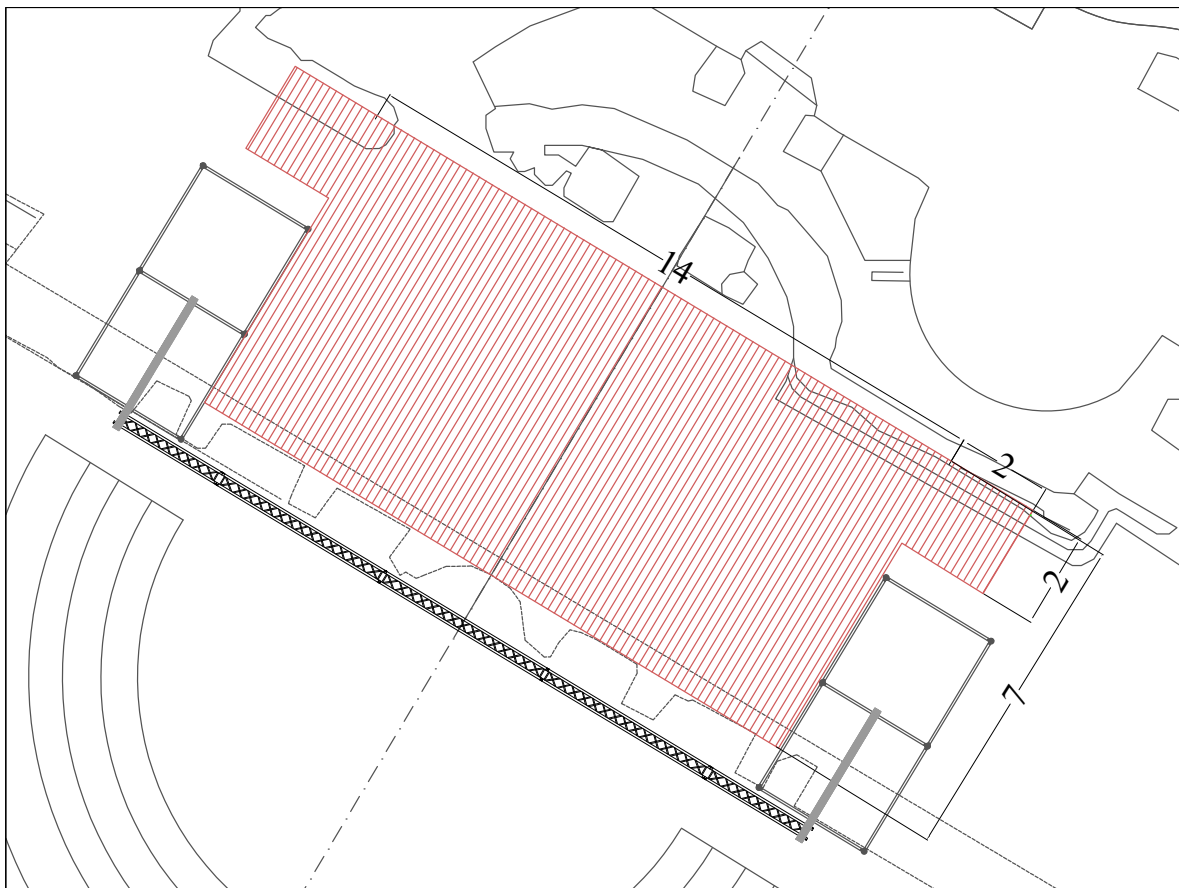
PIANTA PALCOSCENICO
