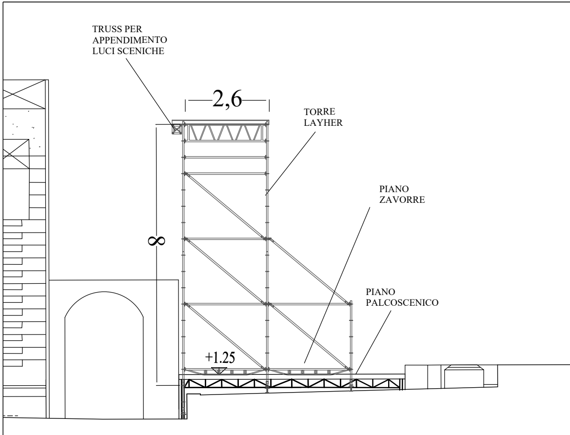
VISTA LATERALE
