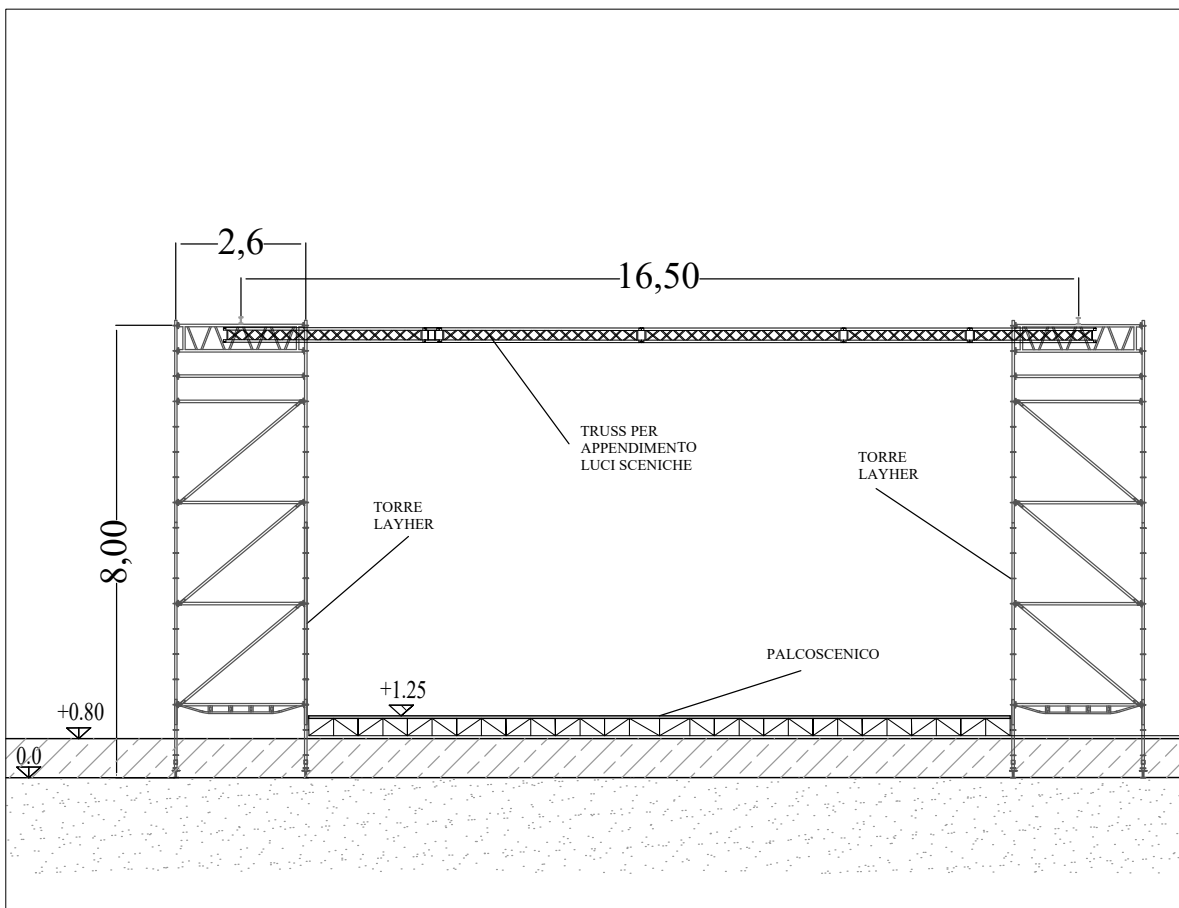
VISTA FRONTALE
